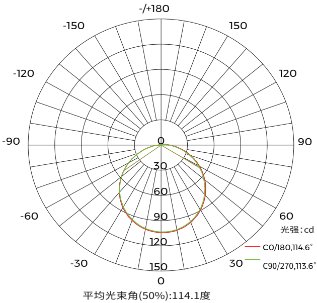
配光曲线
